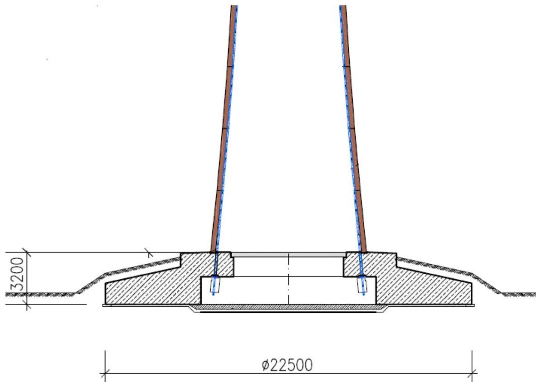
Kuva 4-4. Poikkileikkauskuvaa mahdollisista perustuksista.
