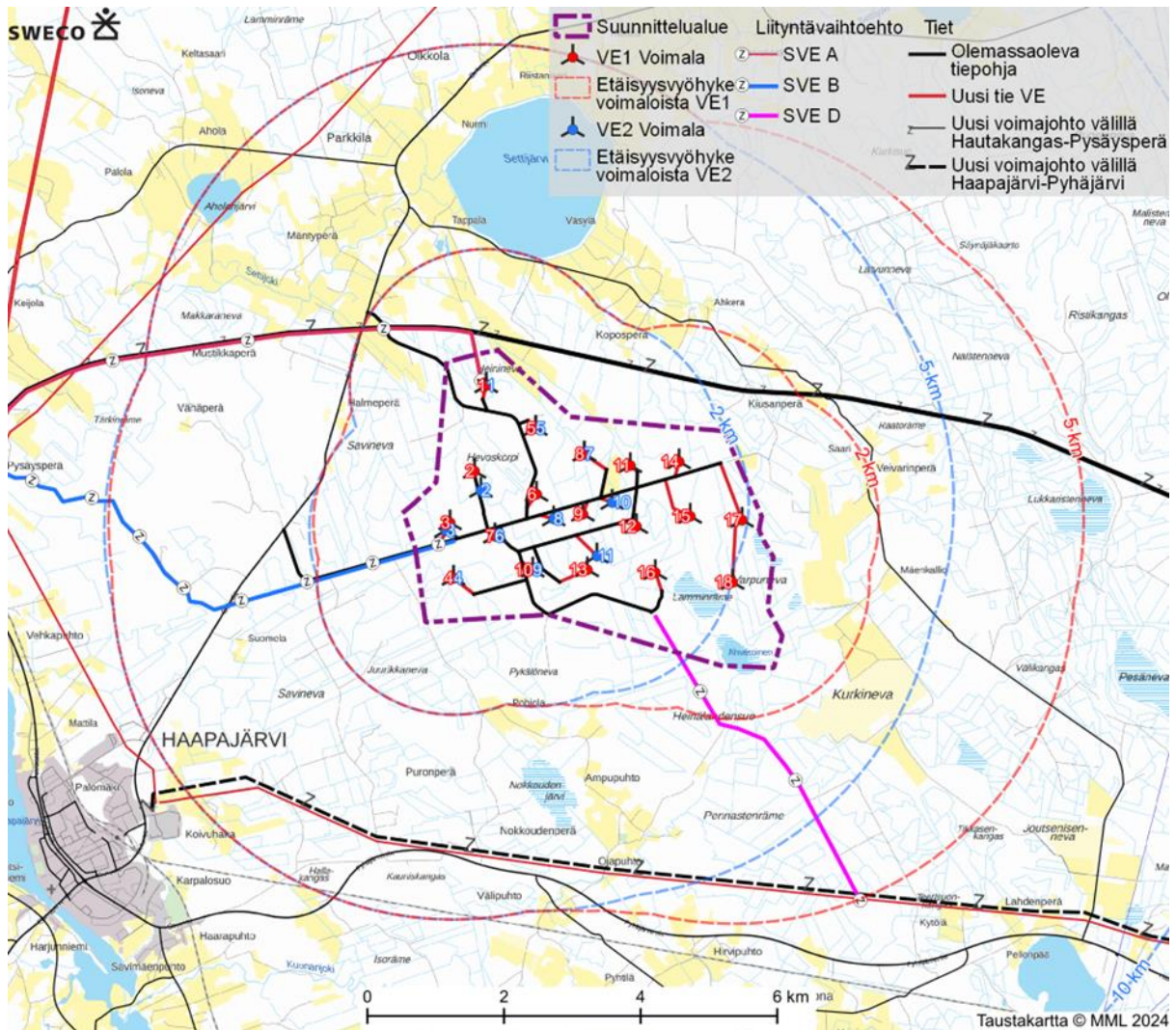
Alustava voimalasijoittelu Korteperän hankealueella. Alueelle rakennetaan 18 voimalaa vaihtoehdossa VE1 tai 11 voimalaa vaihtoehdossa VE2. Kartalla on esitetty myös sähkönsiirron vaihtoehdot.
