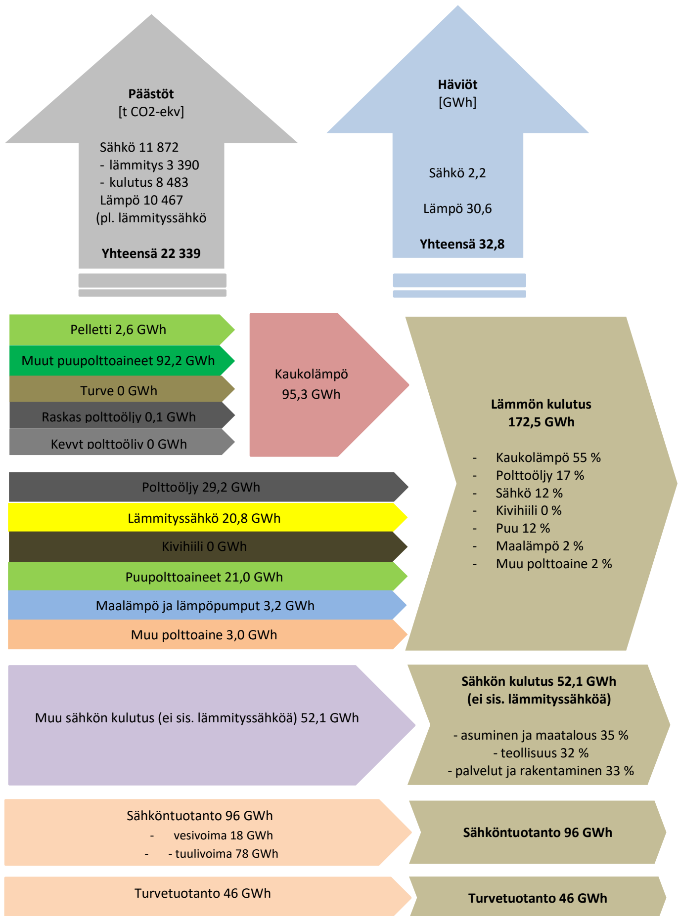
Kuva 18. Haapajärven kaupungin alueen kokonaisenergiatase vuonna 2017.
