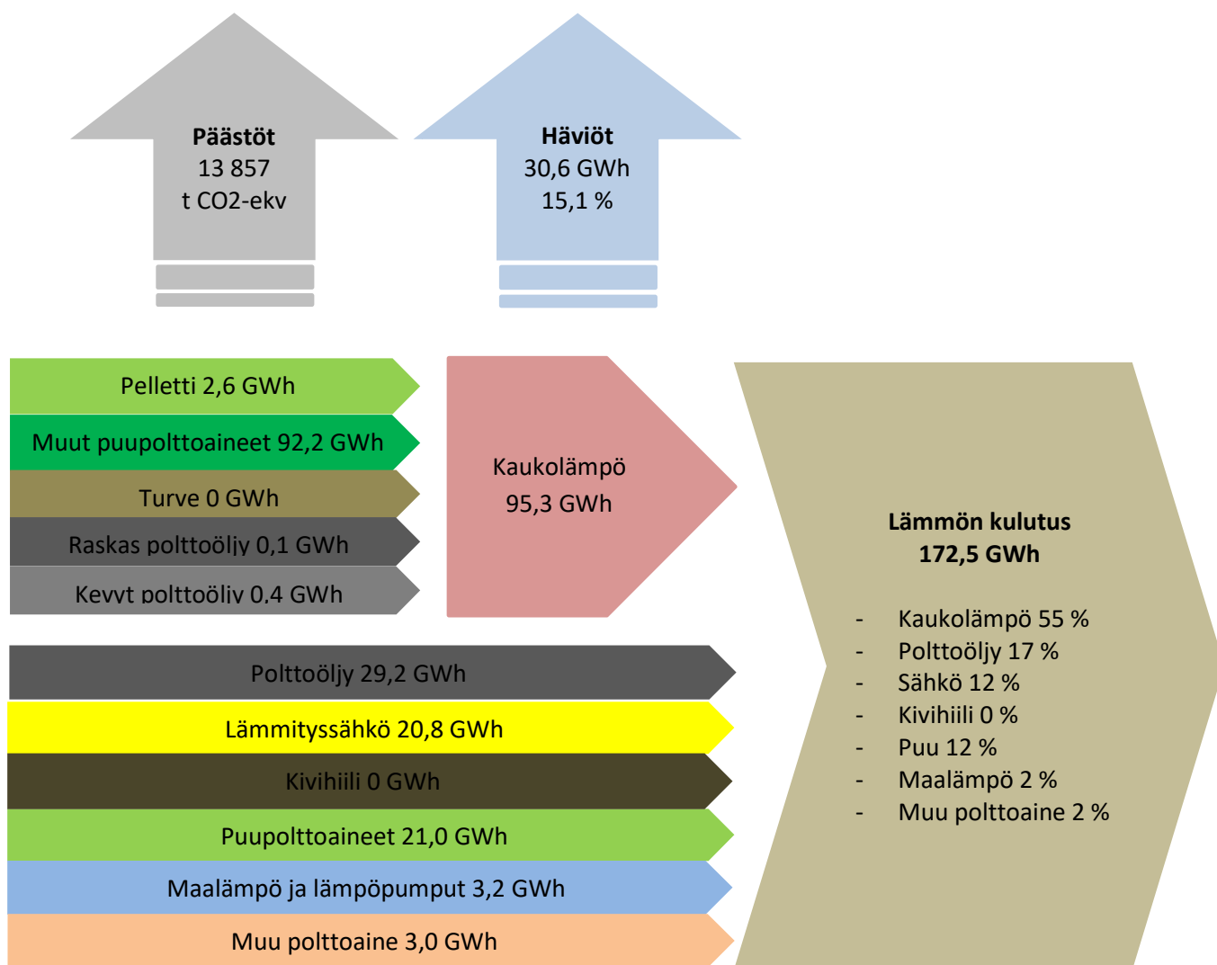
Kuva 15. Haapajärven kaupungin lämpöenergiatase vuonna 2017. Lämmön kulutuslukemat ovat puhdasta kulutusta, häviöt on esitetty kuvan yläosassa erikseen.
